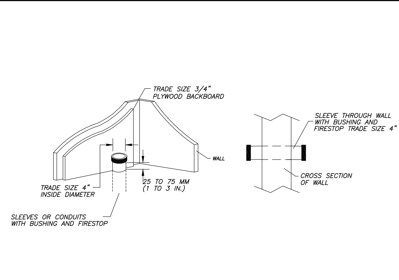
2 SLEEVE/CONDUIT DETAILS
